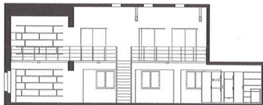
Längsschnitt. Loft im vierten und fünften Stock. Lengtedoorsnede. Vierde en vijfde verdieping van de loft Section longitudinale. Loft quatrième et cinquième étages
